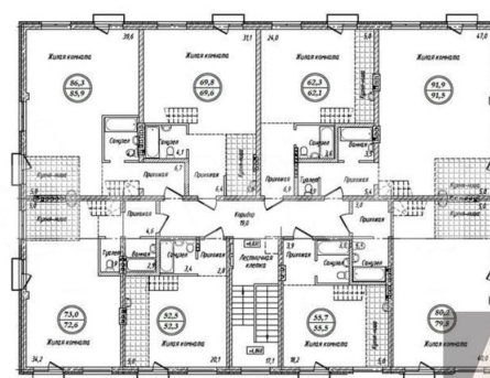
КОРПУС 4 Секция 1 План 3 этажа
