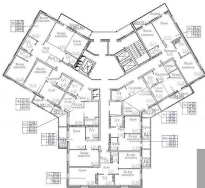
КОРПУС 1 Секция 1 План 2-19 этажей
