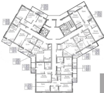
КОРПУС 1 Секция 1 План 20-24 этажей
