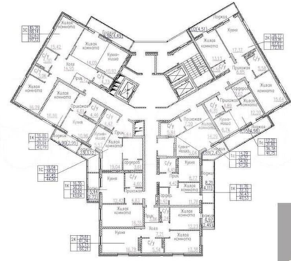
КОРПУС 1 Секция 1 План 2-19 этажей
