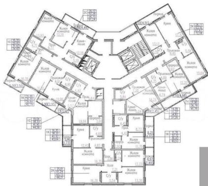
КОРПУС 1 Секция 1 План 20-24 этажей
