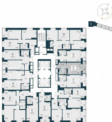
ПЛАН 25-29 ЭТАЖА
