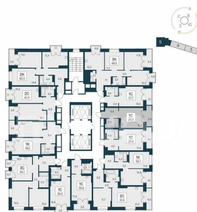
ПЛАН 20, 22-24 ЭТАЖА
